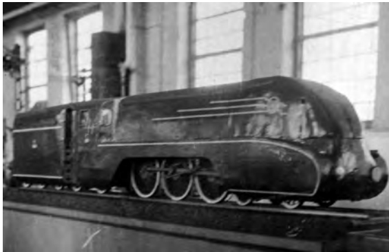
Model parowozu serii Pm36 w otulinie aerodynamicznej, składnica w nieczynnej Parowozowni w Bytomiu, ok. 1956-1957, fot. ze zbiorów Muzeum Techniki NOT w Warszawie
